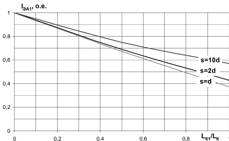
Рис 8. Результаты расчетов по формуле (1.3) для кабеля 240/50 мм 2 в зависимости от соотношения s/d и L_{K1}/L_K .
