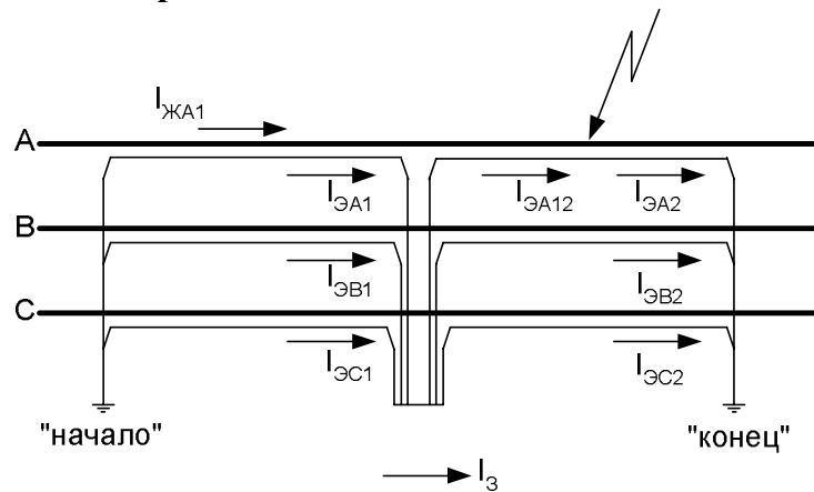
Рис.11. Близкое к «концу» кабеля повреждение изоляции «жила-экран» фазы «А» в группе из трех однофазных кабелей, экраны которых объединены в соединительной муфте.
