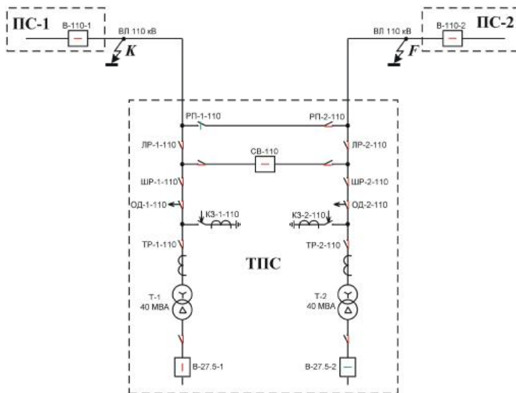
Рис.2. Тяговая подстанция для электроснабжения тяговой сети 25 кВ однофазного тока частотой 50 Гц.
