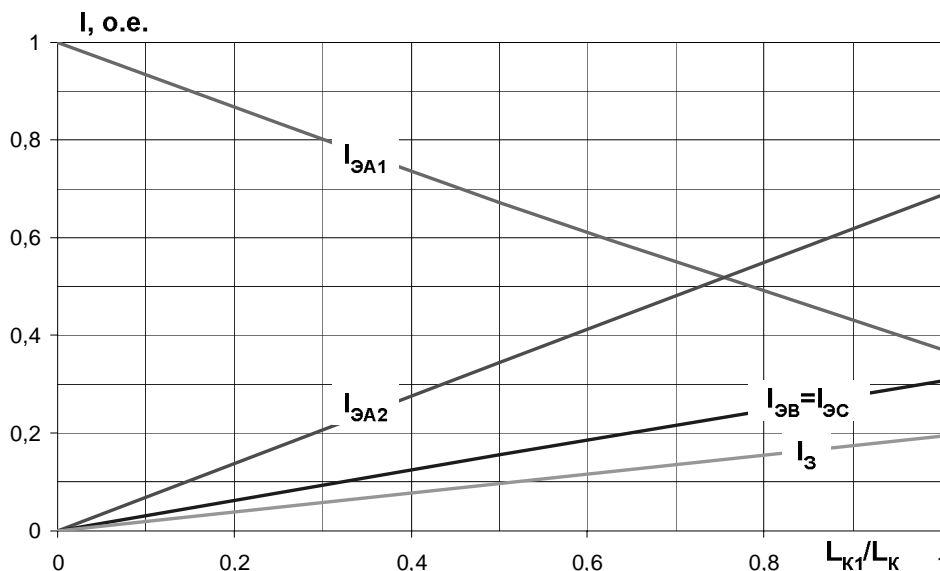
Рис 7. Результаты расчетов по формулам (1.1)-(1.4) при s/d = 1 для кабеля 240/50 мм 2 в зависимости от соотношения L_{К1}/L_K .
