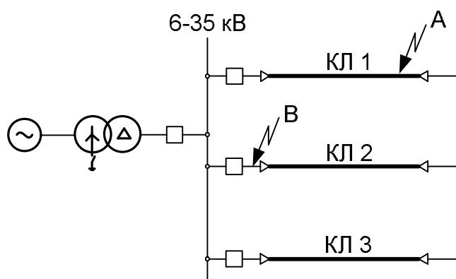
Рис.10. Двойное повреждение изоляции К(1,1) в кабельной сети с изолированной нейтралью.
