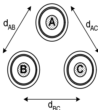
Рис.3. Расположение однофазных кабелей в вершинах равностороннего треугольника.
