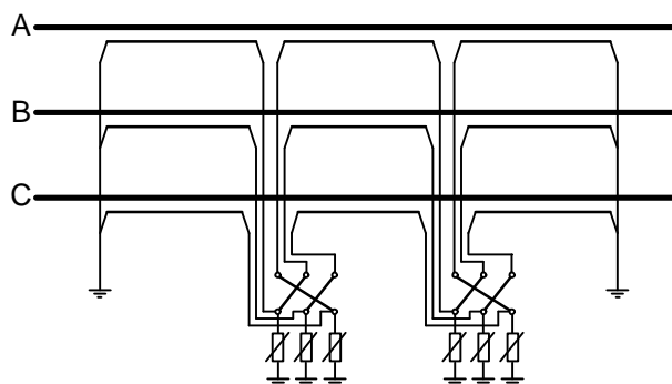
Рис.7. Заземление экранов однофазных силовых кабелей в двух его концах и одновременное применение транспозиции экранов.
