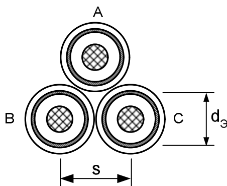
Рис.5. Прокладка трехфазной группы однофазных кабелей в виде сомкнутого треугольника.
