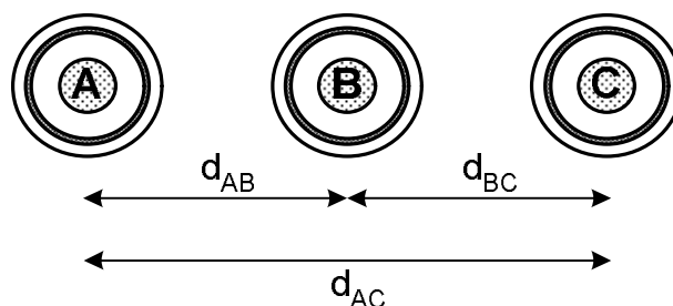
Рис.2. Расположение однофазных кабелей в ряд.
