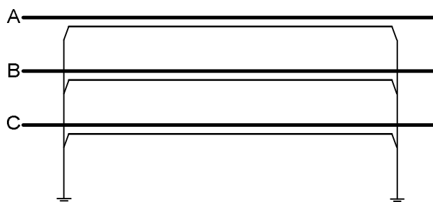
Рис.4. Заземление экранов однофазных силовых кабелей в двух его концах.
