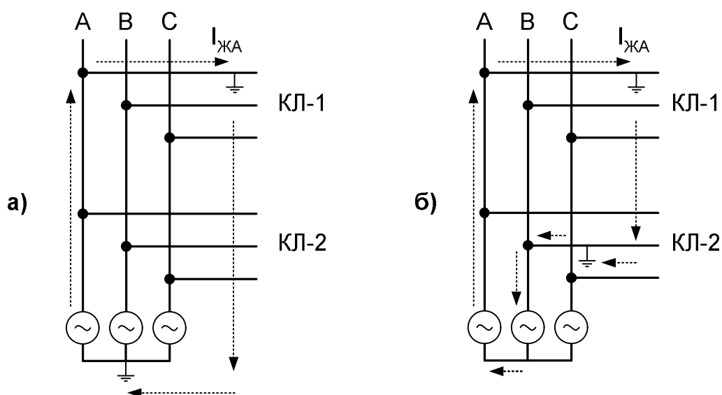
Рис.11. Процессы при повреждениях изоляции: при К(1) в сетях с заземленной нейтралью (а) и при К(1,1) в сетях с изолированной нейтралью (б).
